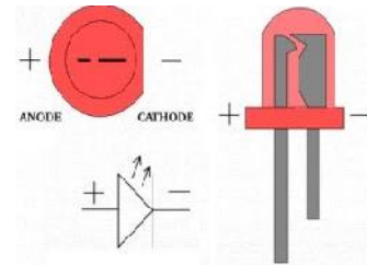
Gambar 3: Simbol dan gambar LED (Sumber: Jago Elektronika, hal 21)
