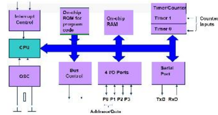
Gambar 1: Diagram blok arsitektur AT89S51
